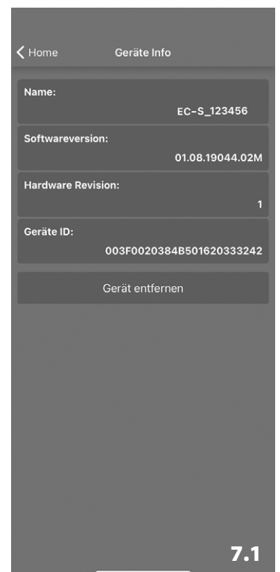
Anzeige der schrauberspezifischen Eigenschaften (Screen 7.1).
